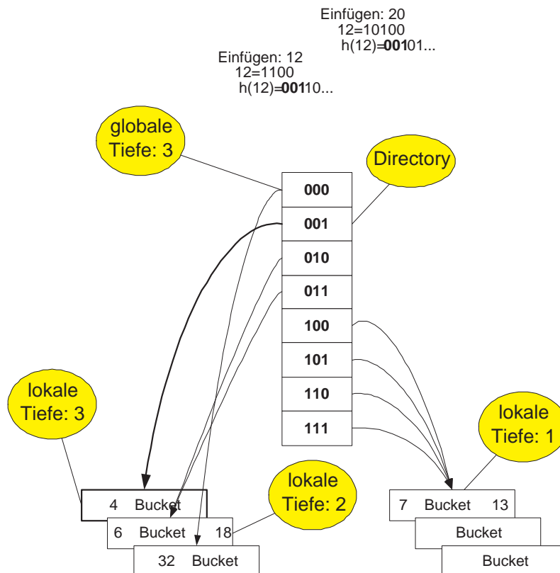
Abbildung 8.14: Illustration des erweiterbaren Hashings: Directory als Array und Überlauf des Buckets für den Präfix 001
