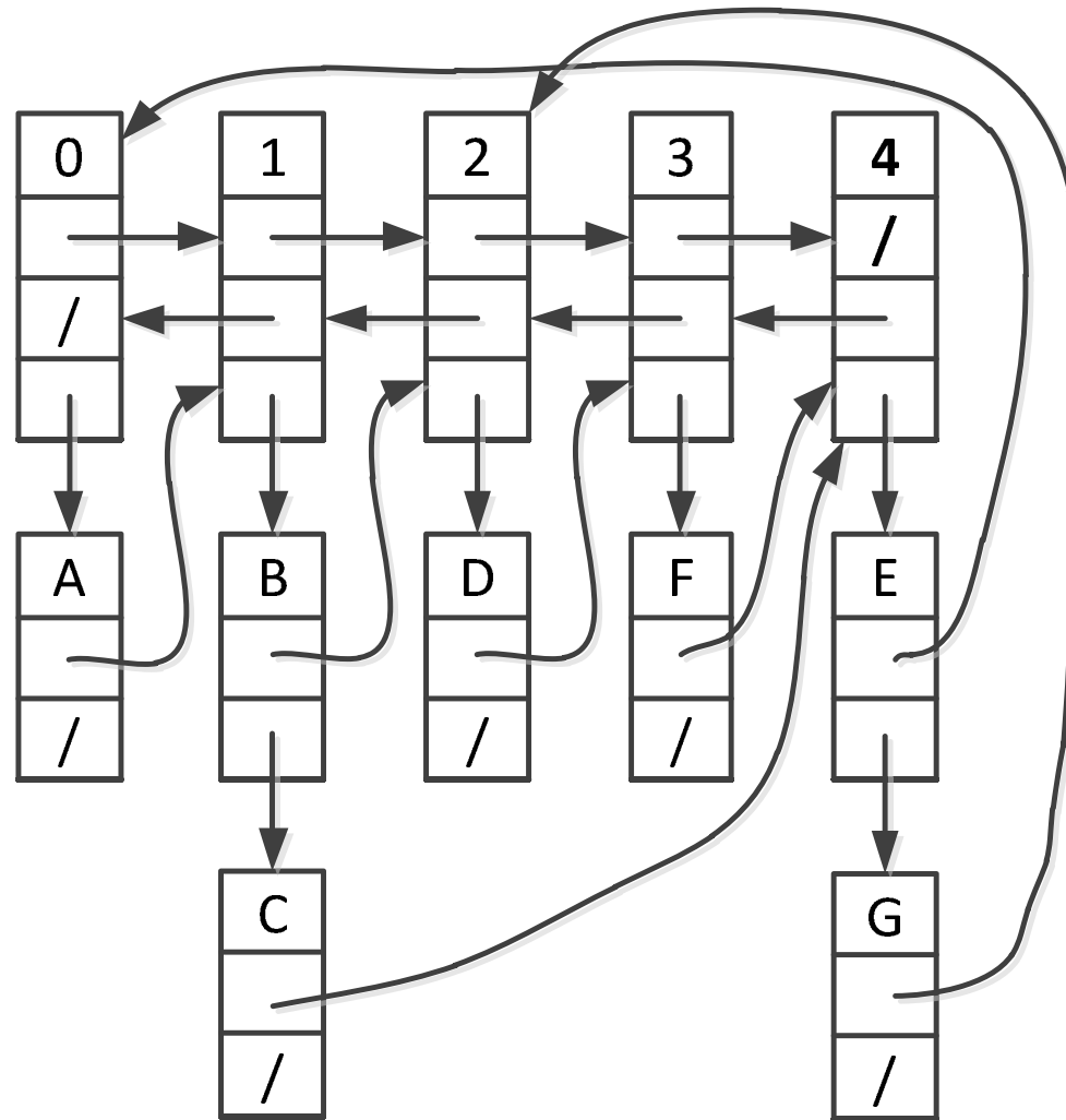
Die vollständig verzeigerte Adjazenzlisten-Struktur
